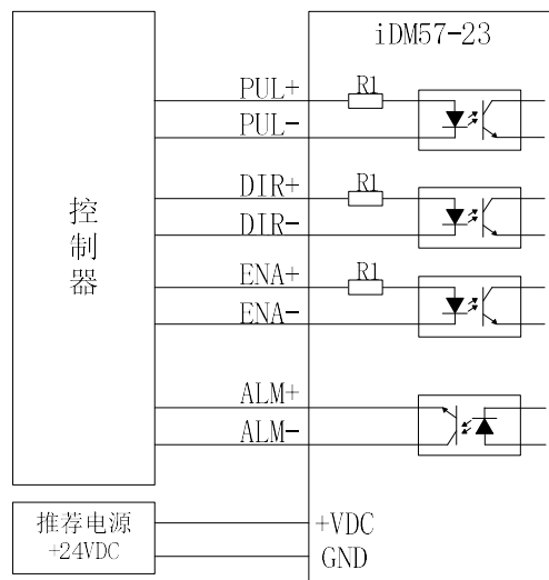
图 3 典型接线图
