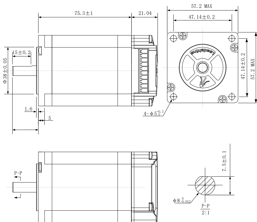
图 1 安装尺寸图
