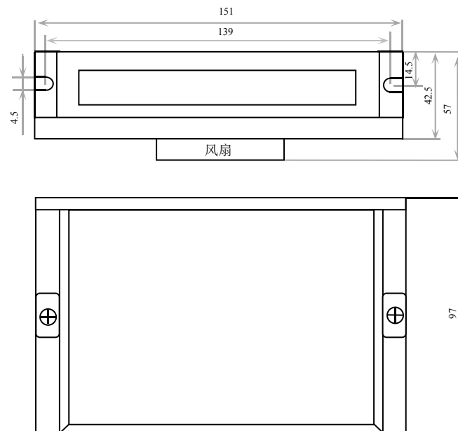
图 1 安装尺寸图（单位：毫米）
