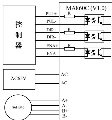
图 6 MA860C (V1.0)配 86 电机典型接法
